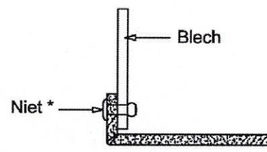
einfache Längsabkantung - verstärkt
