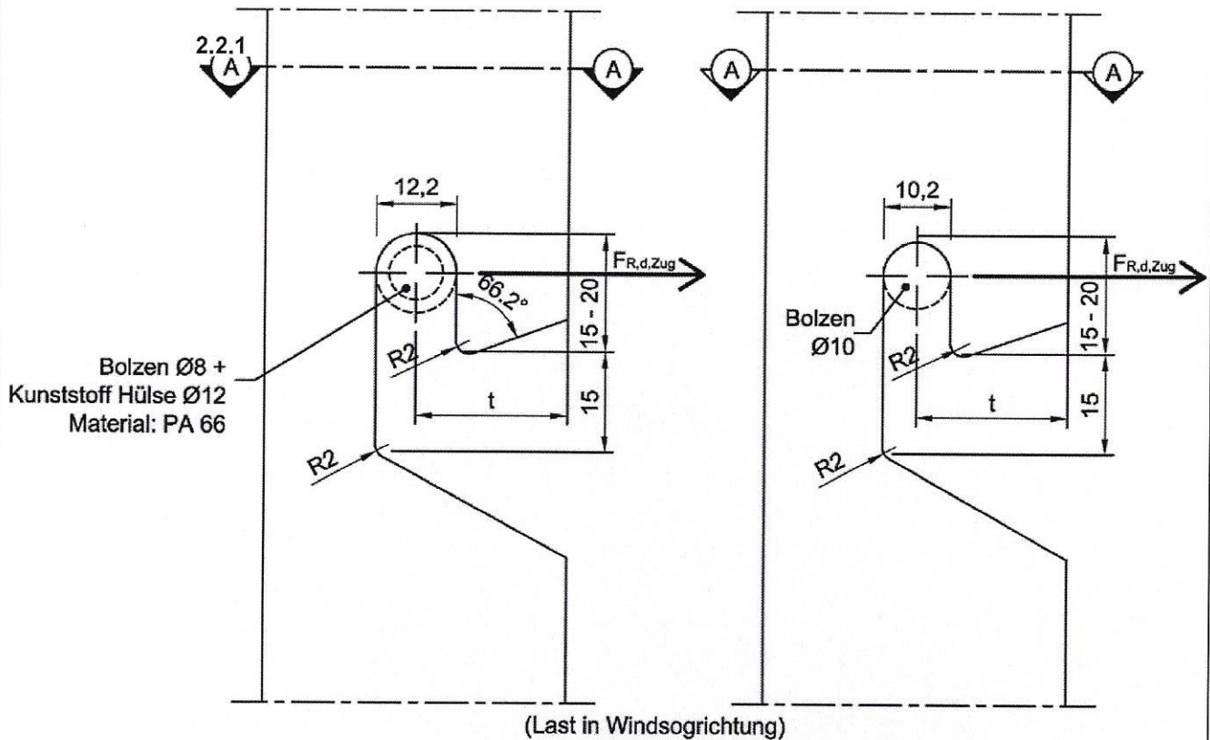
Variante B - Ø10mm Bolzen
