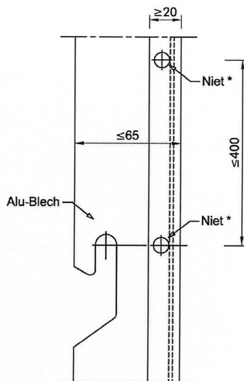
Ausführung 4, Tabelle 1 (Anhang 2) - mit einem Niet je Einhängepunkt
