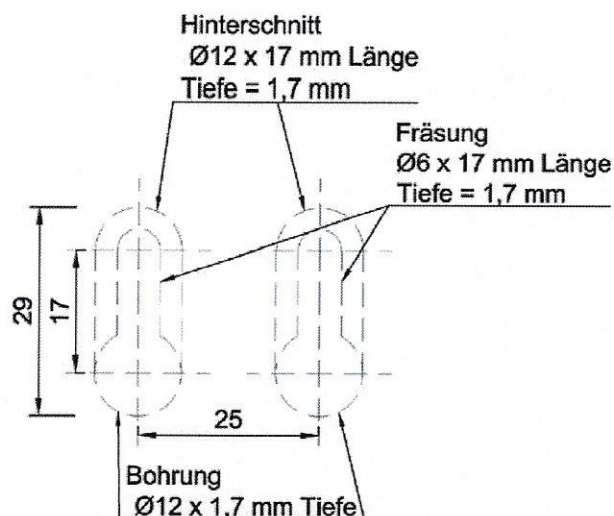
Abmessungen INVISIO-Lochung
