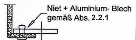
Schnitt A-A - Ausführung 3 + 4
