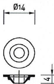
Dichtring Fa-Ze-Di Ø14 mm x 4 mm
