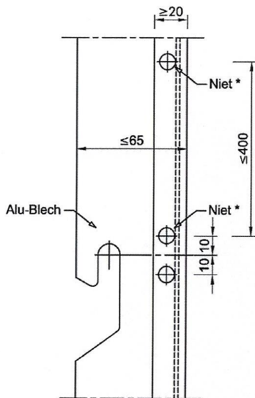
Ausführung 3, Tabelle 1 (Anhang 2) - mit zwei Nieten je Einhängepunkt
