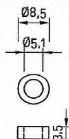
Festpunkthülse Ø8,5 x 3,5 mm - Bohrung Ø5.1 mm
