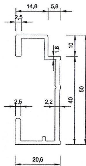
Tragprofil
