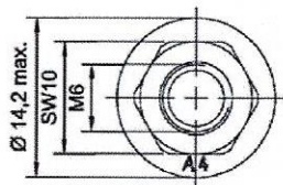
Sperrzahnmutter M6 mit Flansch A4 ähnlich DIN 6923-M6
